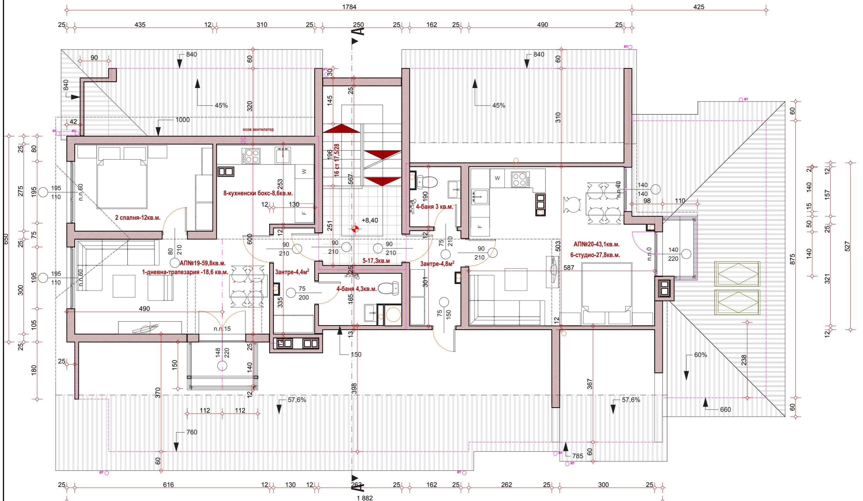
РАЗПРЕДЕЛЕНИЕ НИВО +8.40 М 1:50
