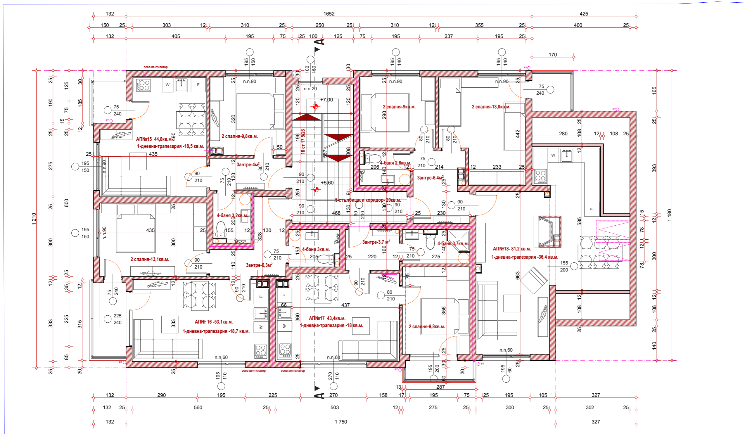
РАЗПРЕДЕЛЕНИЕ НИВО +5,60 М 1:50
