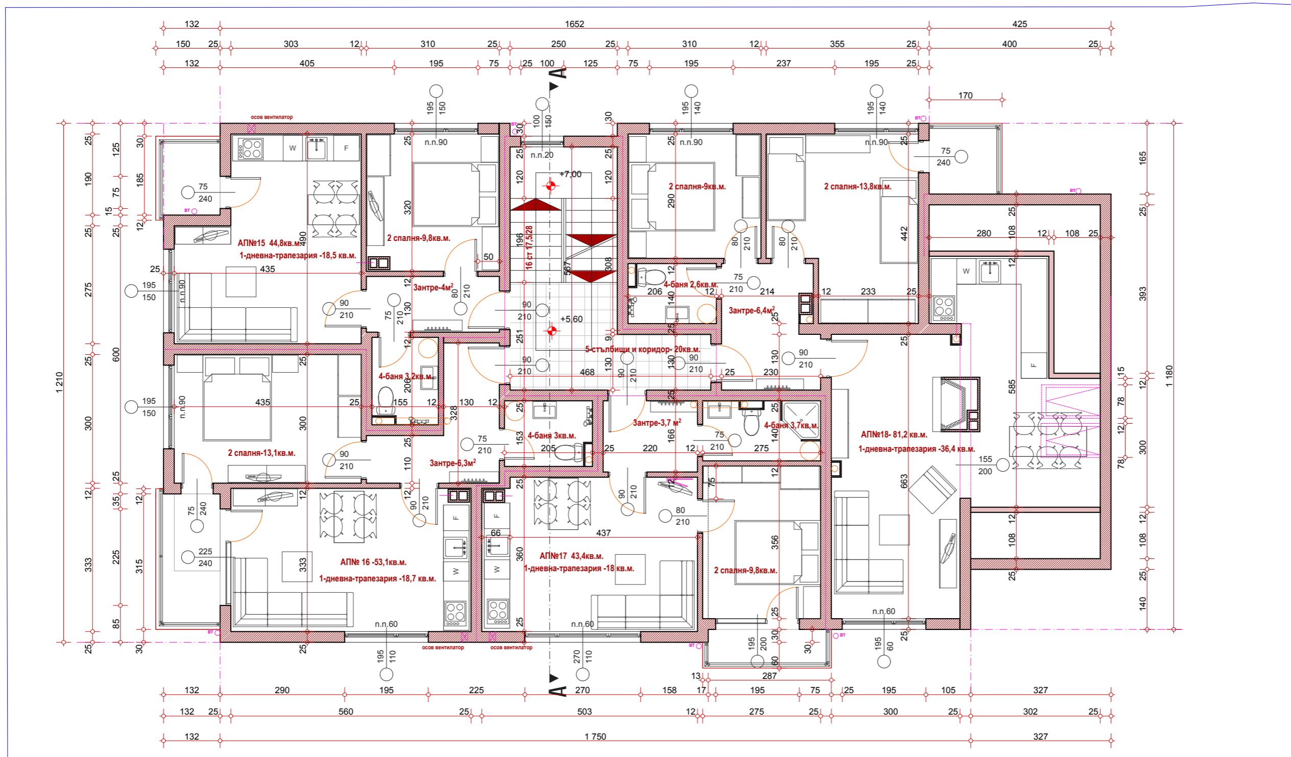
РАЗПРЕДЕЛЕНИЕ НИВО +5,60 М 1:50
