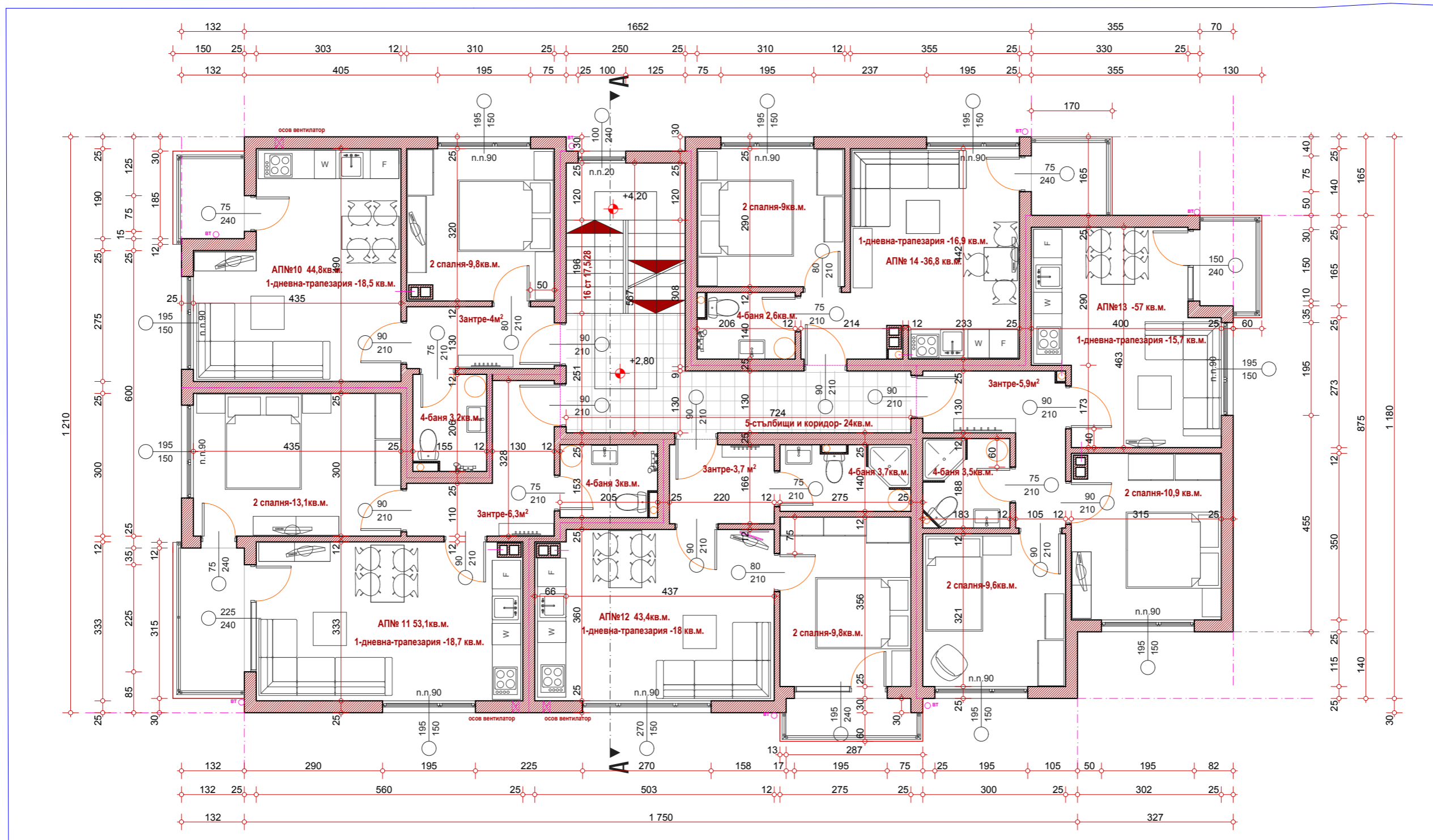
РАЗПРЕДЕЛЕНИЕ НИВО +2,80 М 1:50
