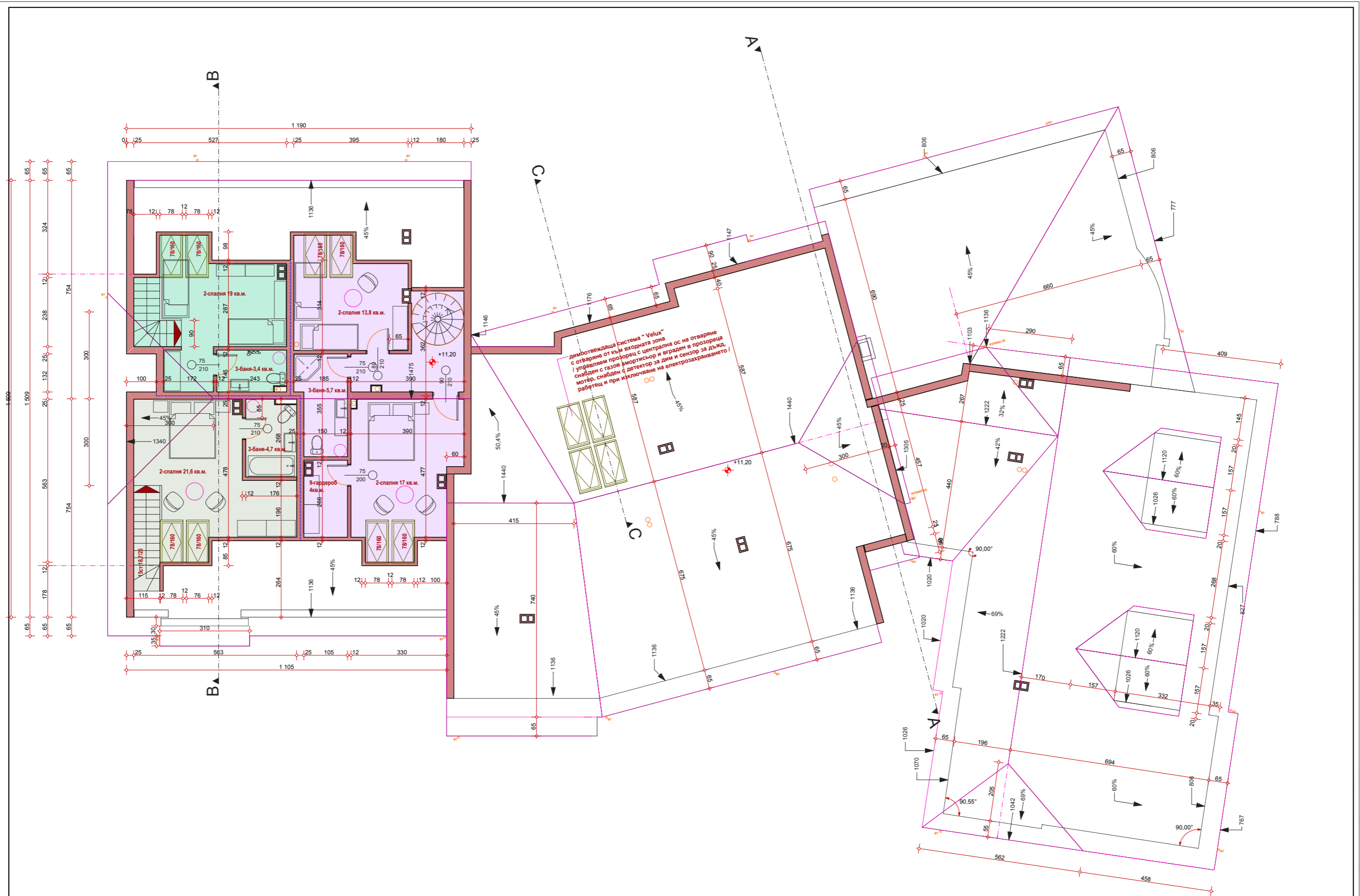
РАЗПРЕДЕЛЕНИЕ НИВО ±0.00 ПО ПОВЕРХНОСТИ НА 1:50
