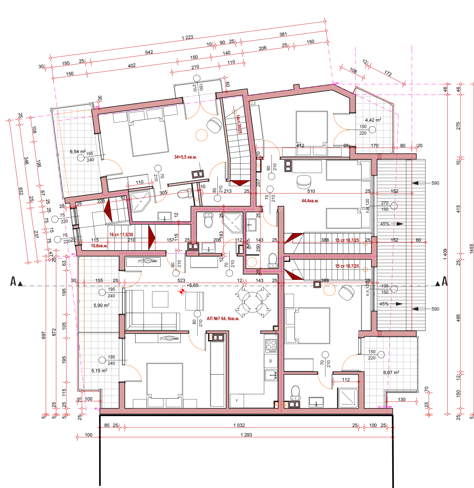
РАЗПРЕДЕЛЕНИЕ МАНСАРДА КОТА +5,60 ВАРИАНТ
