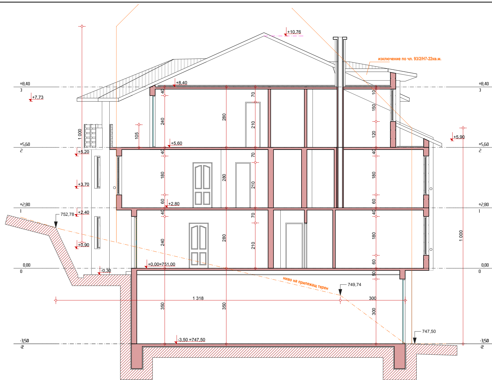
РАЗРЕЗ А-А М 1:50
