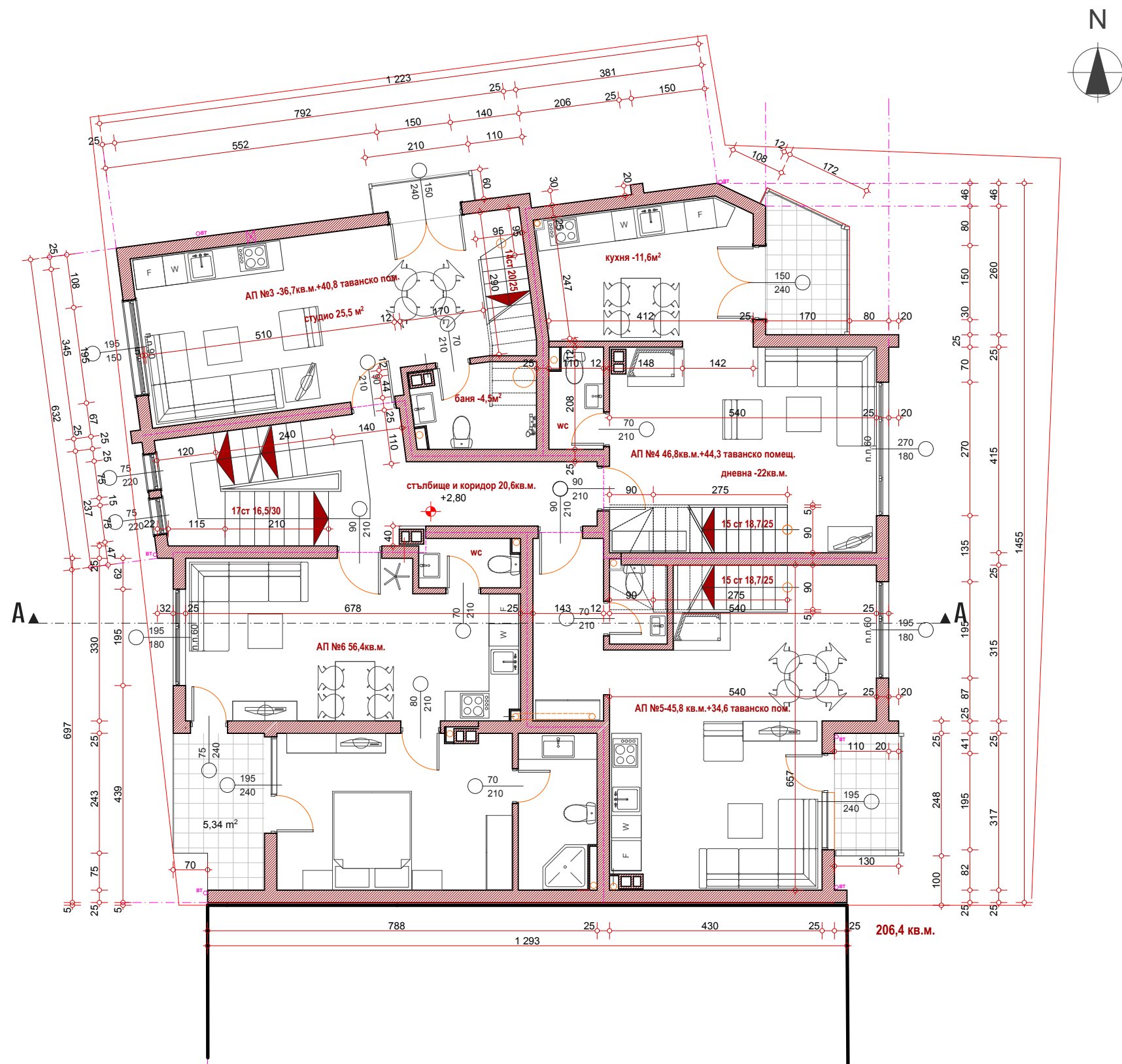
РАЗПРЕДЕЛЕНИЕ 2 ЕТ. КОТА 2,50 М 1:50-ВАРИАНТ
