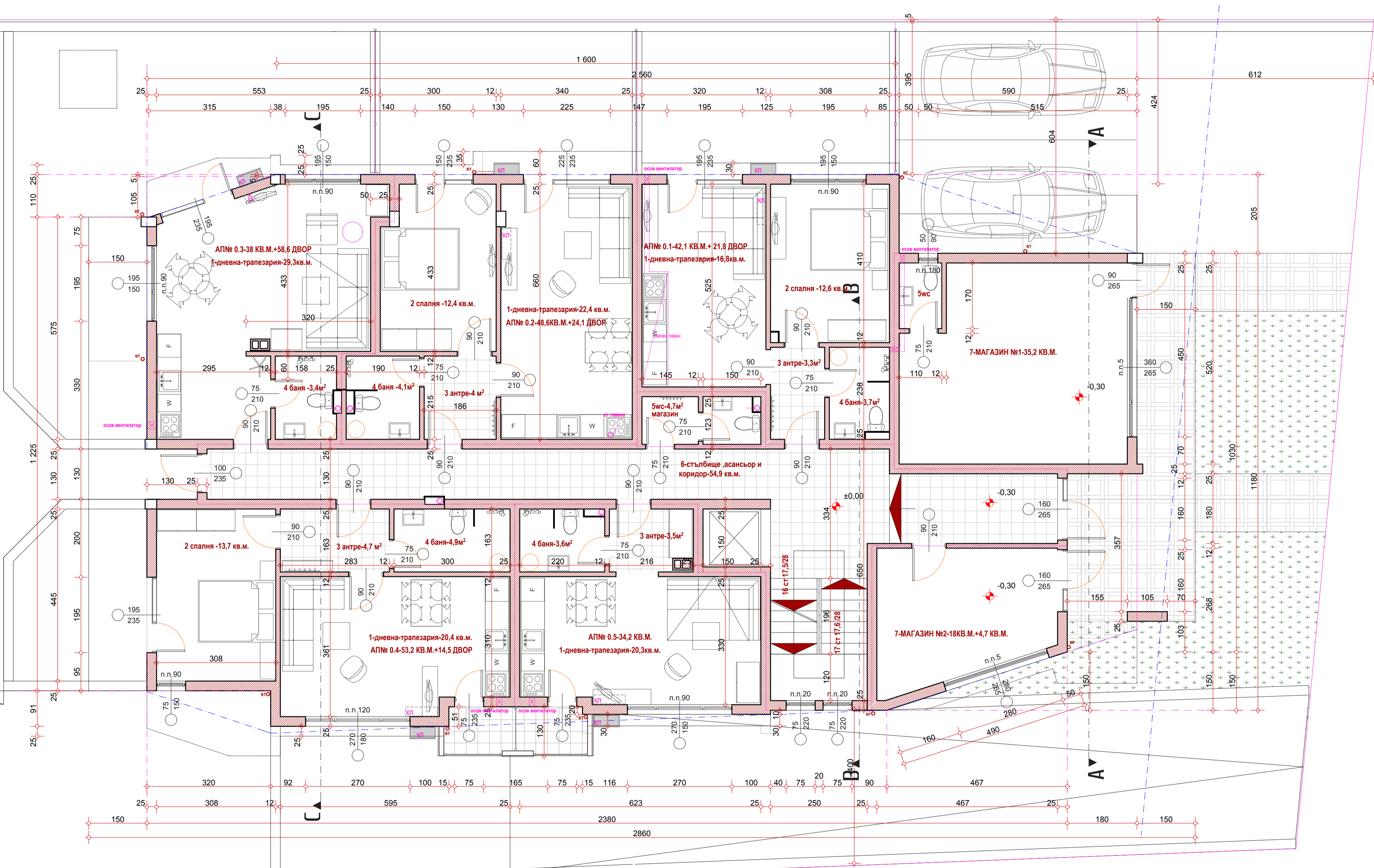
РАЗПРЕДЕЛЕНИЕ ПАРТЕР М 1:50
