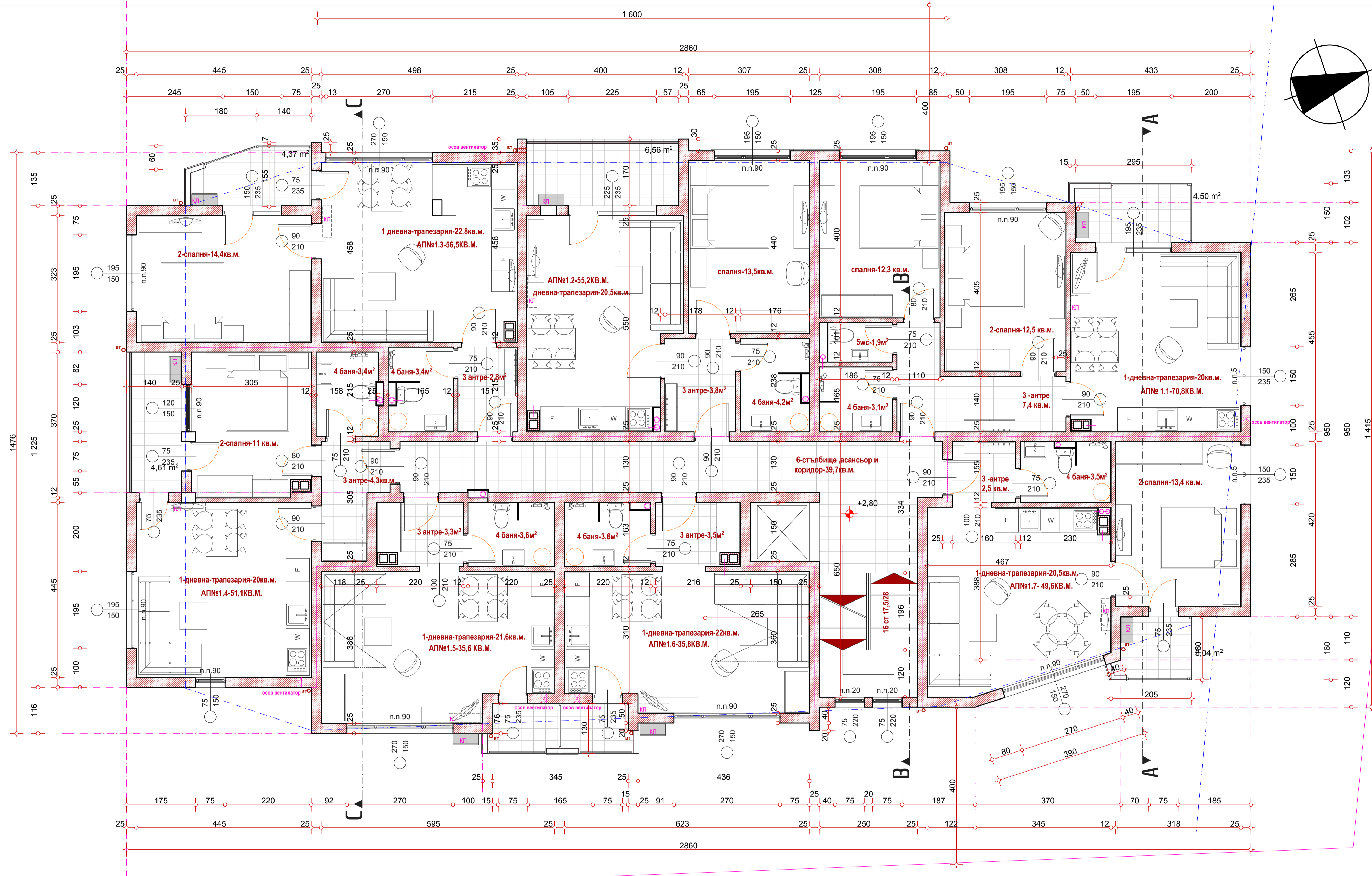
РАЗПРЕДЕЛЕНИЕ 1 ЕТАЖ М 1:50
